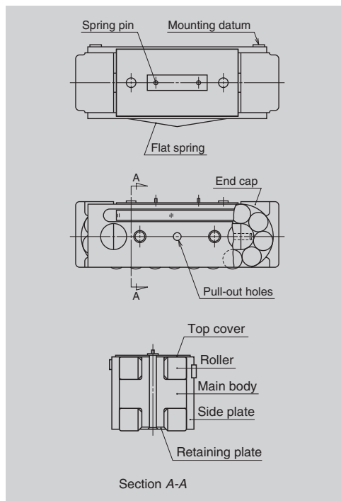
Fig. 1 Roller pack
